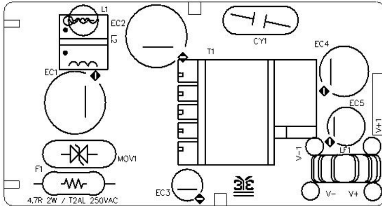
TOP OVERLAY
