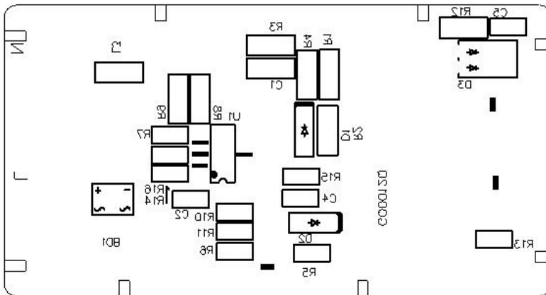
BOTTOM OVERLAY
